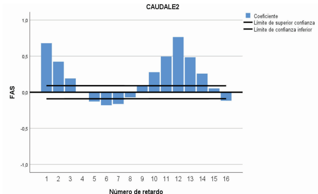
Figura 6. Función de autocorrelación. Fuente: Autores
