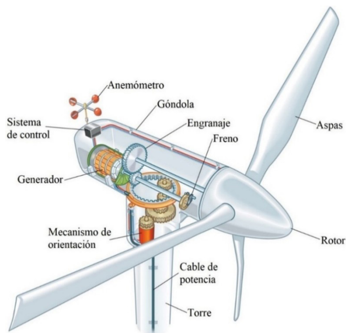
Figura 2. Partes turbina eólica (Sosapanta, 2020).
