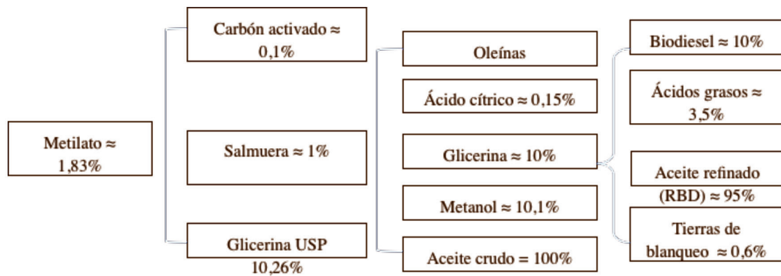
Fig. 3 Composiciones de los productos obtenidos en la fabricación de biodiesel a partir de aceite de palma.
