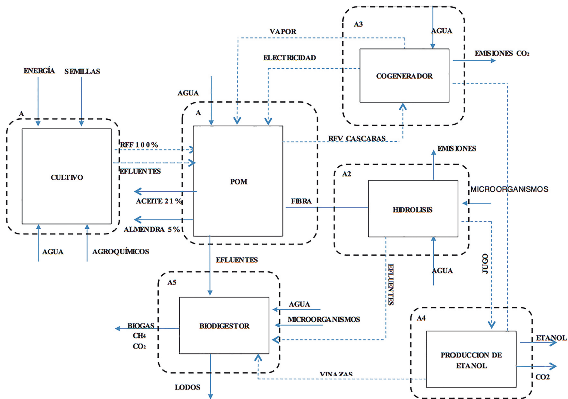
Fig. 7 Diagrama esquemático de entradas y salidas del sistema.
