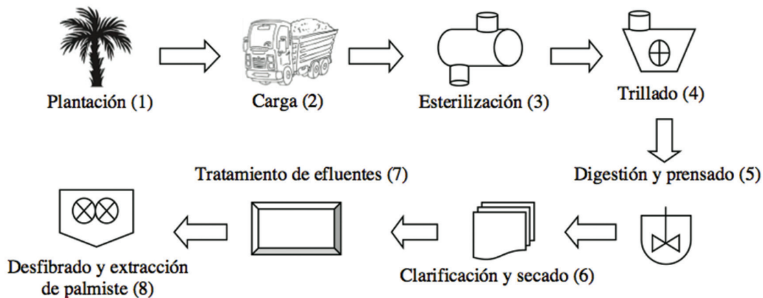
Fig. 2 Descripción del proceso tradicional de extracción del aceite de palma.
