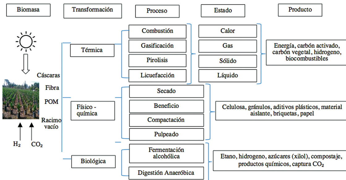
Fig. 5 Alternativas para el uso de la biomasa de la palma de aceite.
