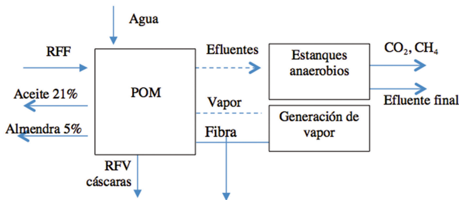
Fig. 6 Escenario general de las plantas extractoras en la que los productos principales son únicamente aceite de palma y almendra.
