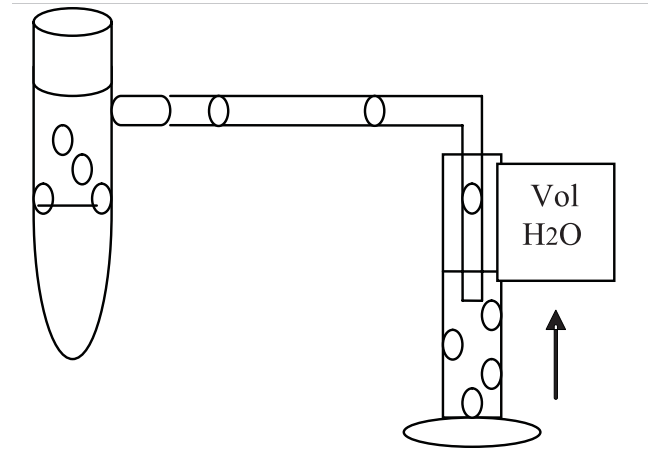
Figura 4. Representación esquemática del desplazamiento de agua por burbujeo.
