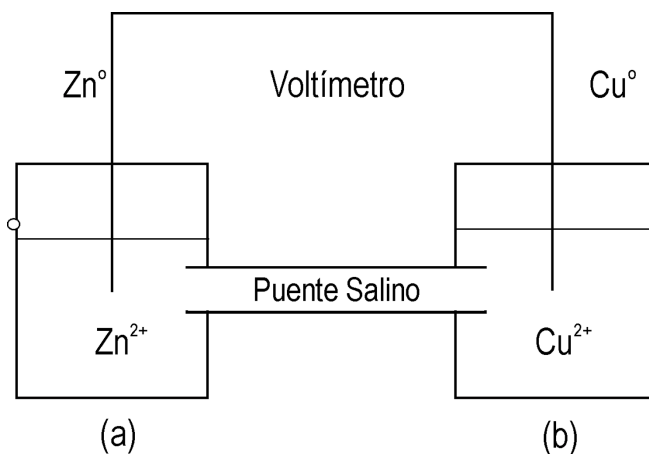
Figura 1. Pila voltaica. Los recipientes (a) y (b) contienen soluciones acuosas de iones Zn^{2+} e iones Cu^{2+} , respectivamente; en los cuales se encuentran inmersos electrodos de Zn^0 y de Cu^0 . Los electrones fluyen desde el electrodo de Zn^0 hasta los iones de Cu^{2+} del recipiente (b). La energía producida es medida mediante el voltímetro. El puente salino conecta los dos recipientes y mantiene el equilibrio de iones.
