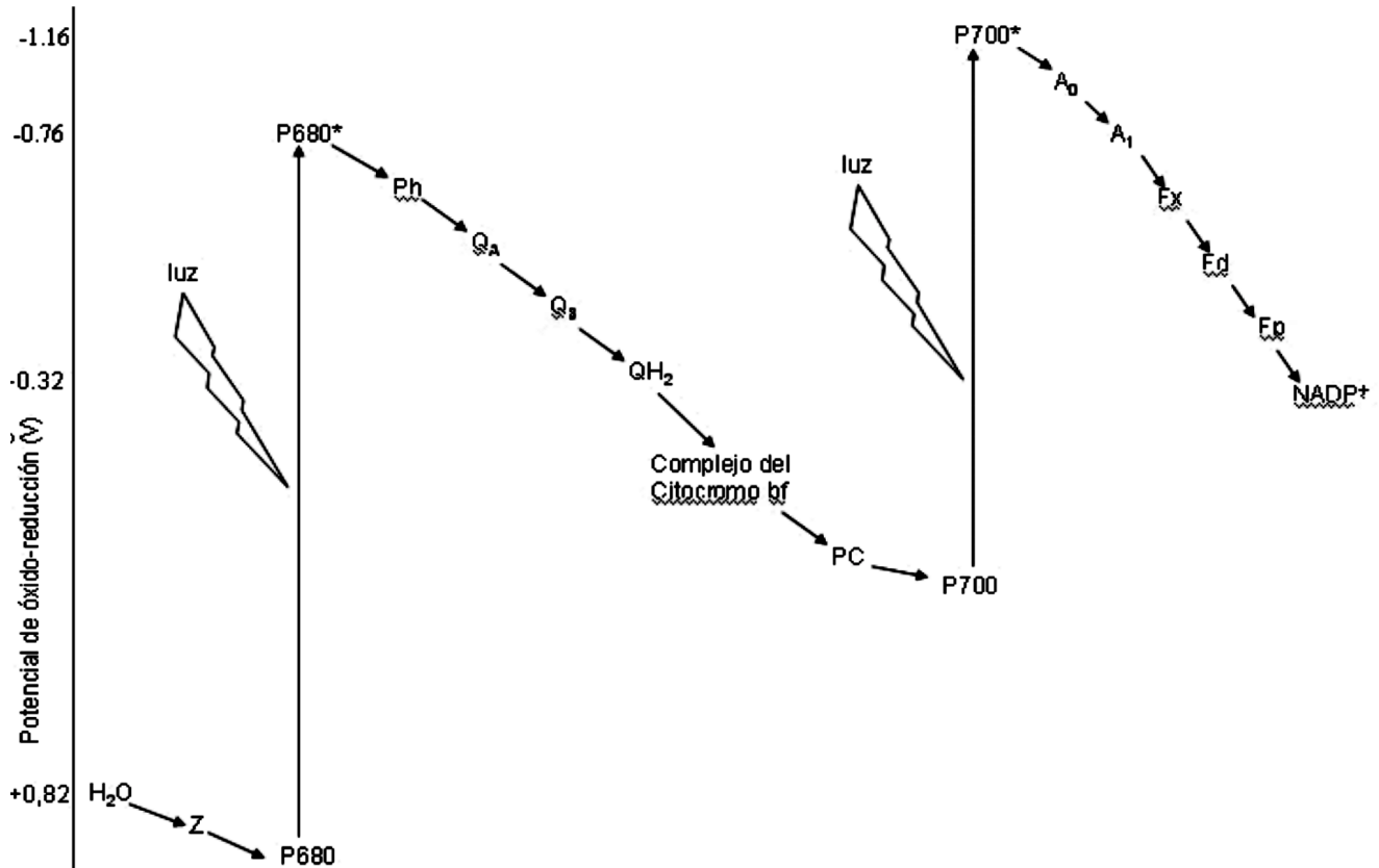
Figura 2. Fotosíntesis oxigénica en una planta. El eje vertical hacia la izquierda del diagrama, representa la variación en los potenciales de óxido-reducción que van desde los muy positivos (abajo) hasta las muy negativos (arriba); de tal manera que la transferencia de electrones es termodinámicamente favorable (con liberación de energía útil) si se realiza desde una molécula que se encuentra en la parte superior del diagrama, hasta una molécula que se encuentra en la parte inferior del mismo. El donador inicial de electrones es el \text{H}_2\text{O} y el aceptor final es \text{NADP}^+ . Note que el flujo de electrones total no sería termodinámicamente favorable por cuanto el potencial de óxido-reducción del \text{H}_2\text{O} es muy positivo (alta afinidad por los electrones) con respecto al potencial del \text{NADP}^+ que es muy negativo (baja afinidad por los electrones). Sin embargo, la incidencia de la radiación solar, proporciona la energía suficiente para que el pigmento P680 pase a un estado activado ( \text{P680}^* ) con un potencial de óxido-reducción tan negativo, que es capaz de generar un flujo de electrones termodinámicamente favorable entre los transportadores de electrones Ph, \text{Q}_A , \text{Q}_B , \text{QH}_2 , Complejo del citocromo \text{b}_6 y PC. El mismo mecanismo de activación y transporte ocurre en el pigmento P700, permitiendo la reducción final del \text{NADP}^+ , utilizando los transportadores de electrones \text{A}_0 , \text{A}_1 , Fx, Fd y Fp.
